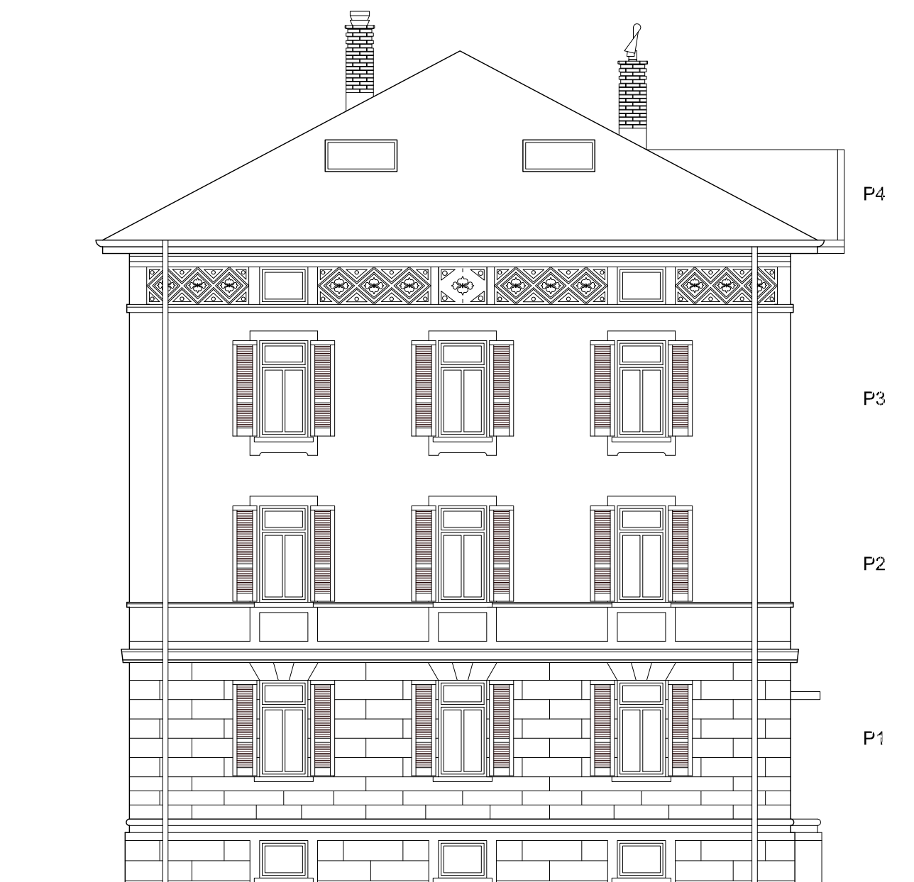
PROSPETTO NORD
