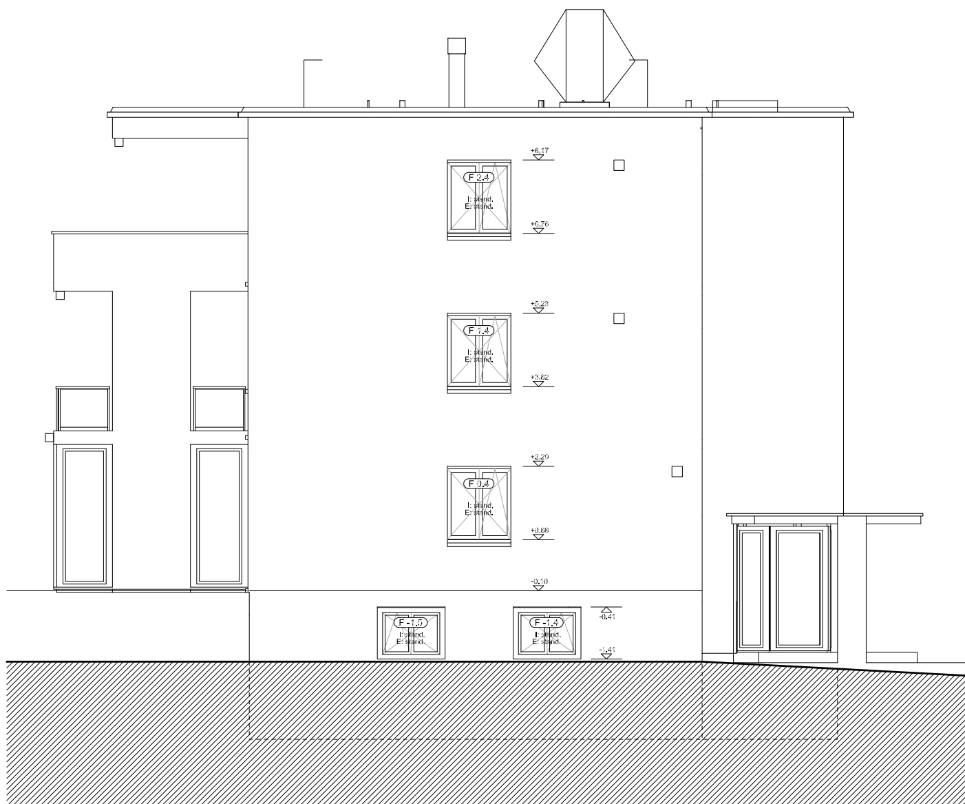
PROSPETTO SUD
